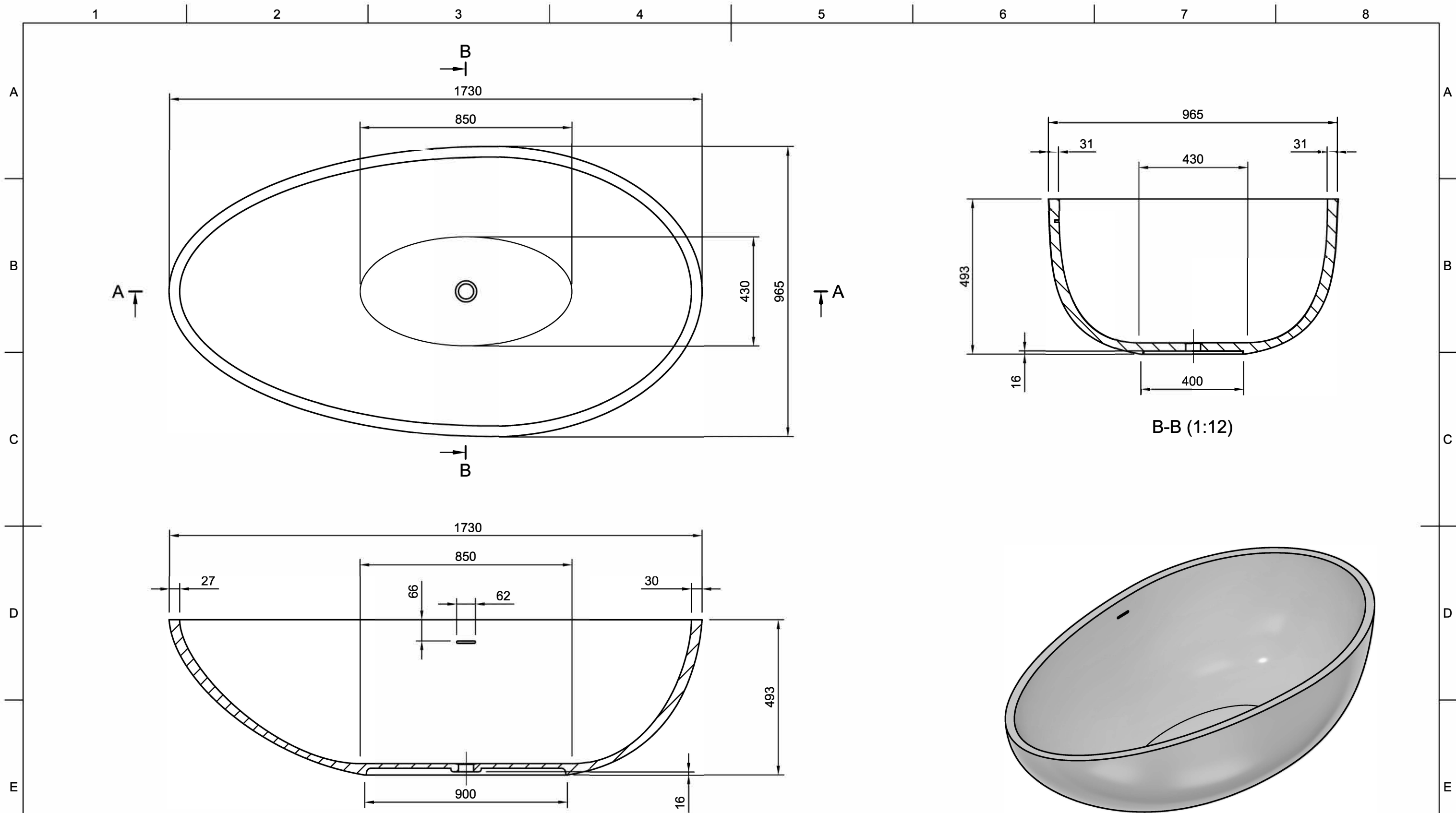
A-A (1:12)
